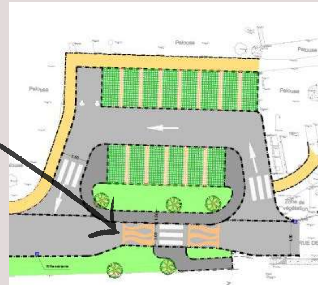
Croisillons envisagés de part et d'autre des passages piétons délimitant la zone de partage
