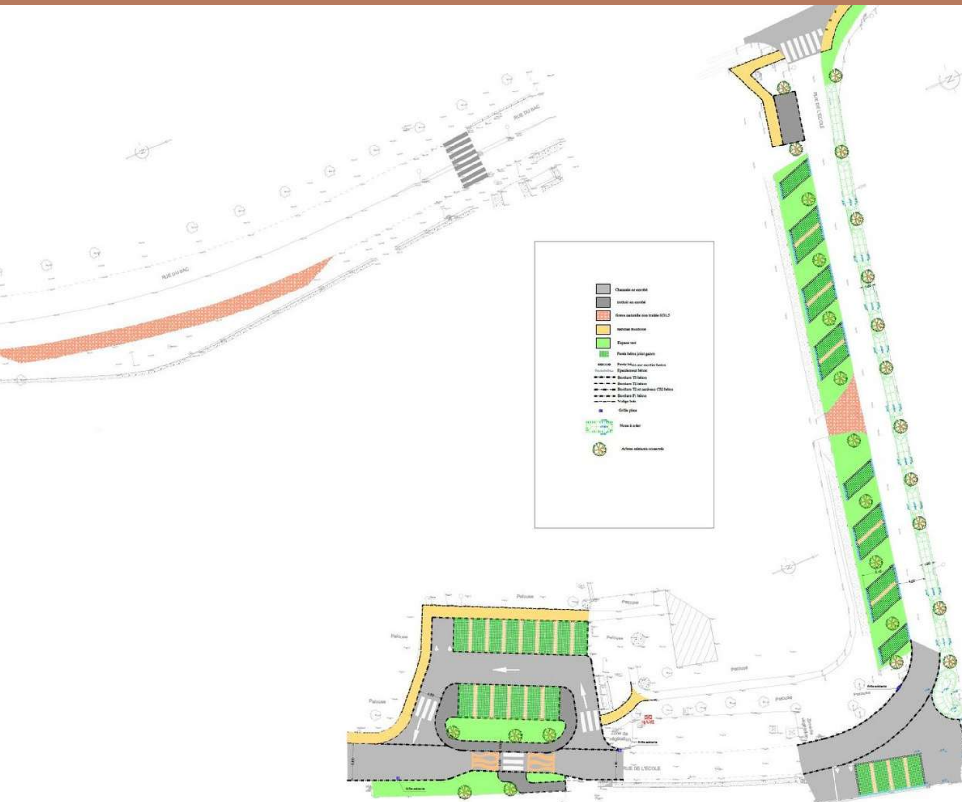
Plan d'esquisse du centre bourg
